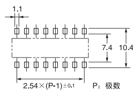
印刷基板加工尺寸 (TOP VIEW)
